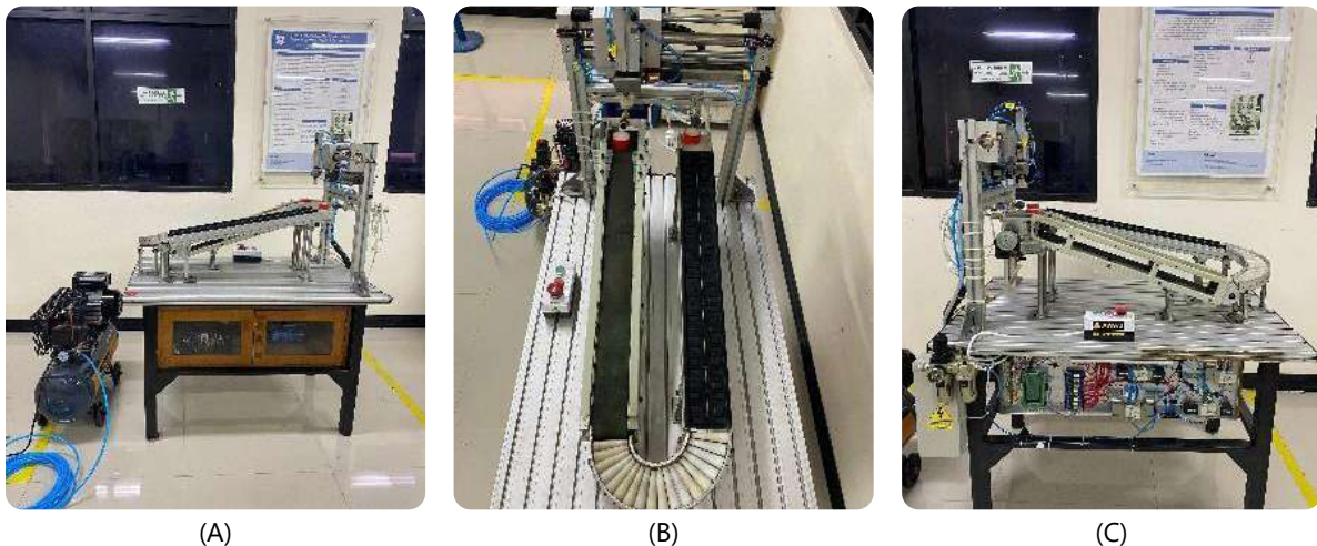
Gambar 2: (A,B,C) Prototipe pemindah barang dengan sistem pneumatik menggunakan mikrokontroler Arduino.
