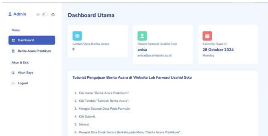
Gambar 9: Halaman dosen
