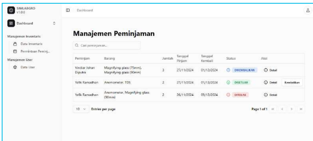
Gambar 5: Status Peminjaman Alat dan Bahan SIMLABGRO-UG
