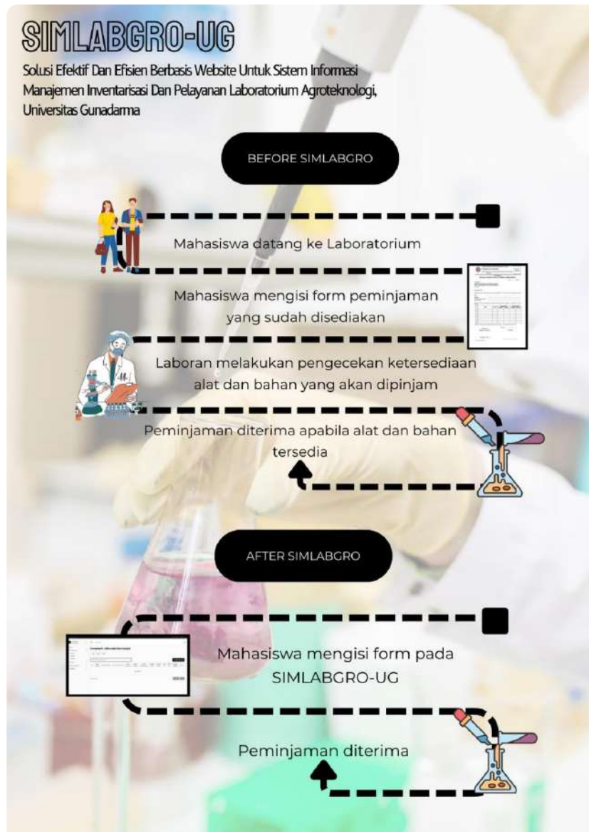
Gambar 1: Infografis SIMLABGRO-UG
